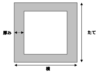
角パイプ断面寸法
